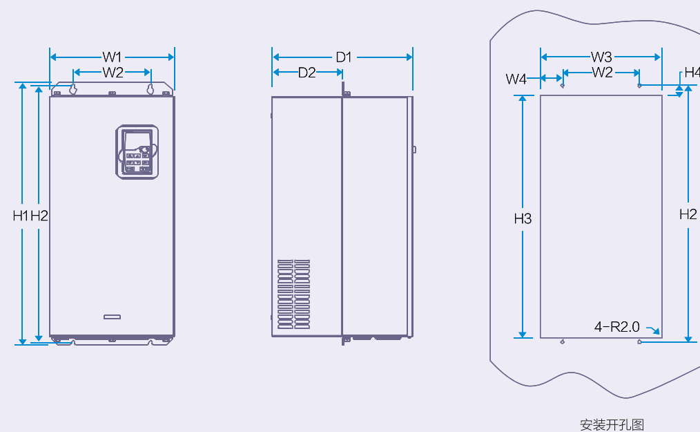
37~110kW法兰安装示意图
