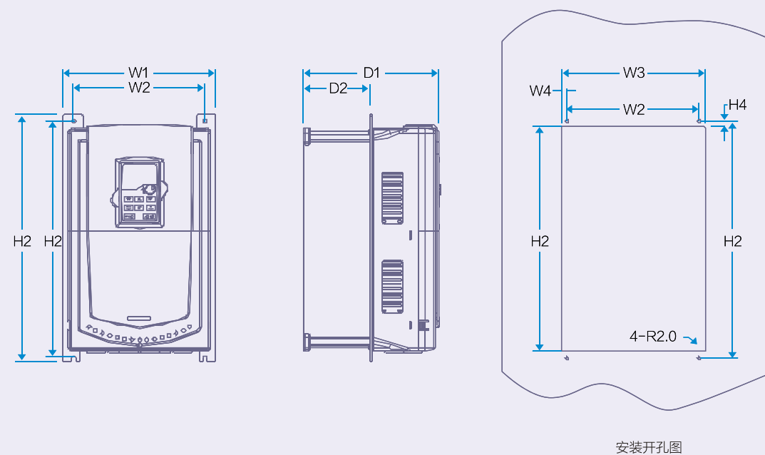
1.5~30kW法兰安装示意图
