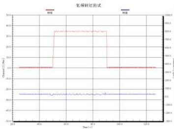
转矩与转速
