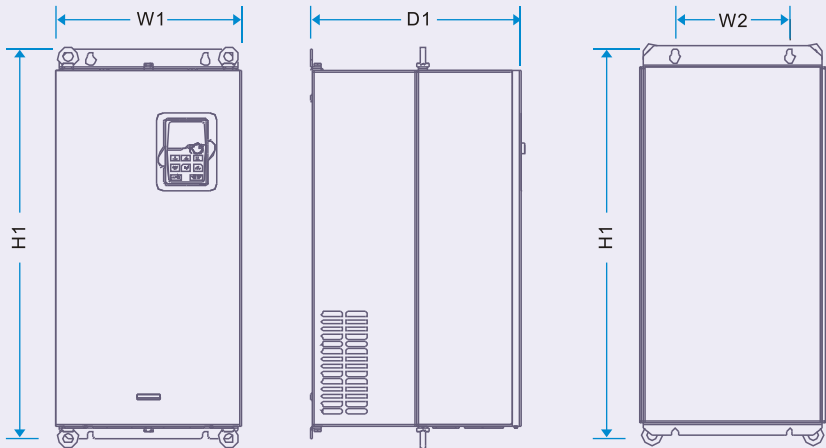
37~110kW壁挂安装示意图
