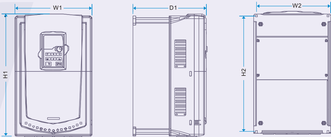
1.5~30kW壁挂安装示意图
