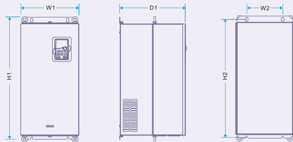
132~200kW壁挂安装示意图
