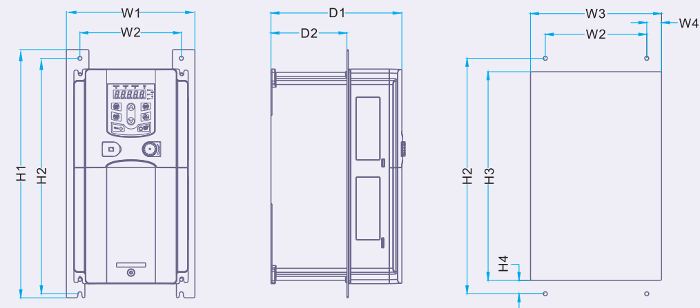
18.5~30kW法兰安装示意图
