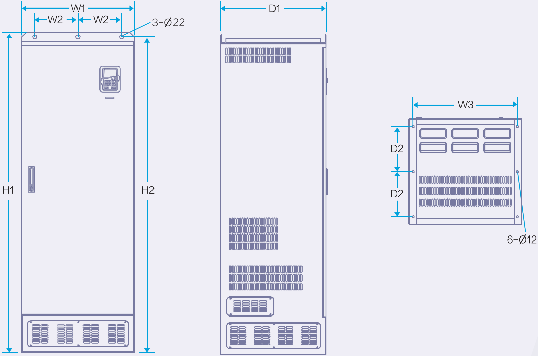
350kW~500kW落地安装示意图
