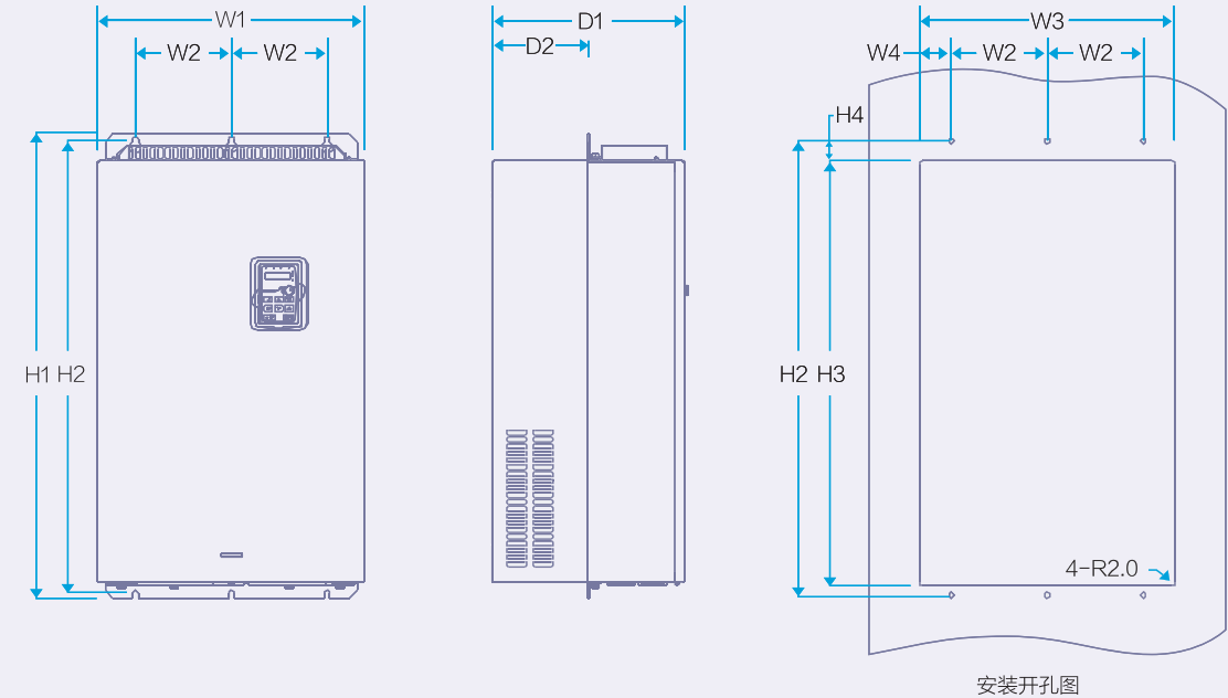
132~200kW法兰安装示意图
