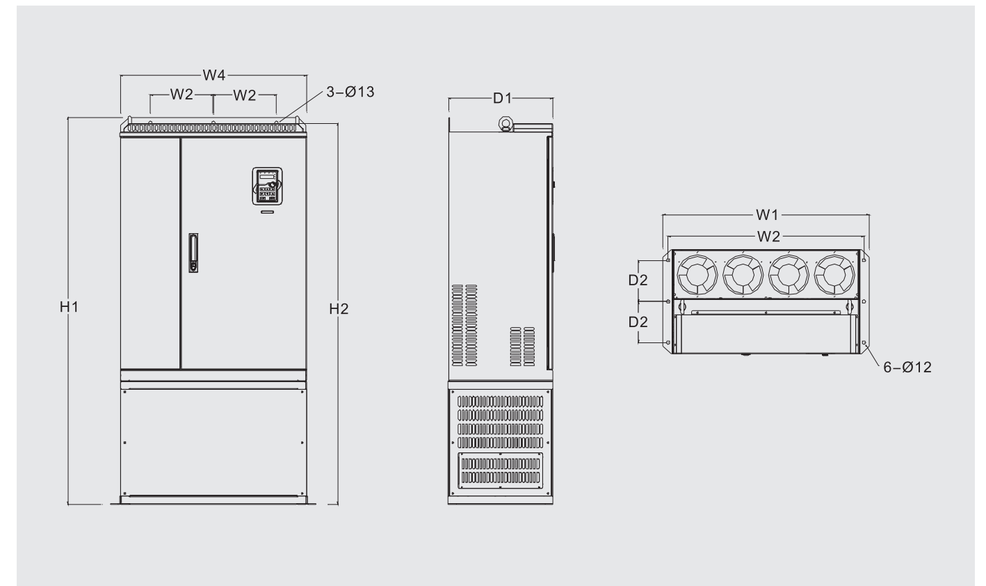
■ 380V 220~315kW ( 660V 250~350kW ) 落地安装示意图
