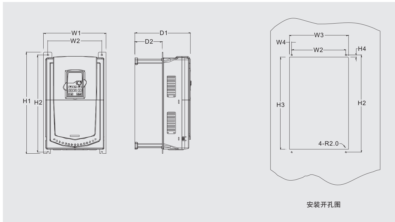
■ 380V 1.5~30kW法兰安装示意图
