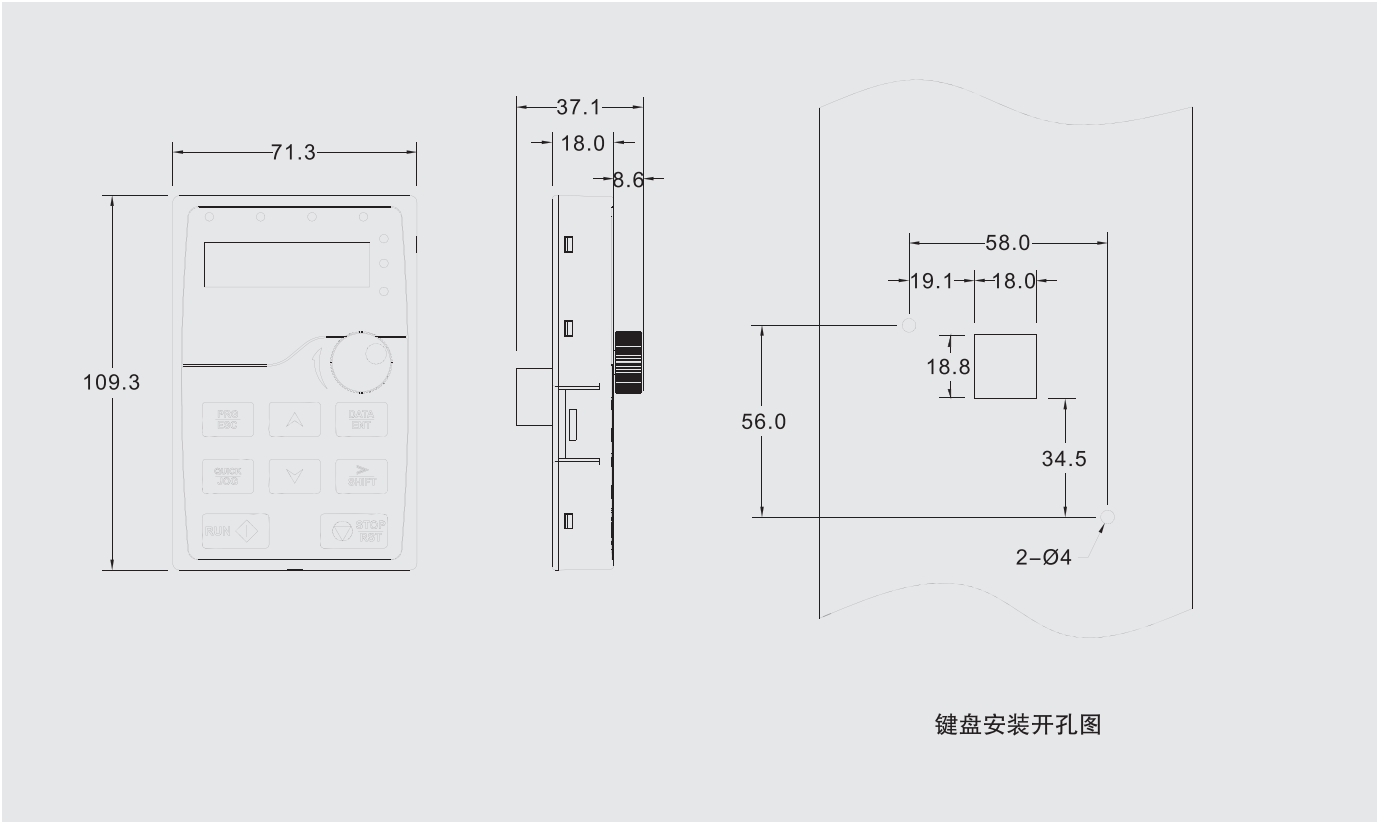
键盘外形尺寸图
