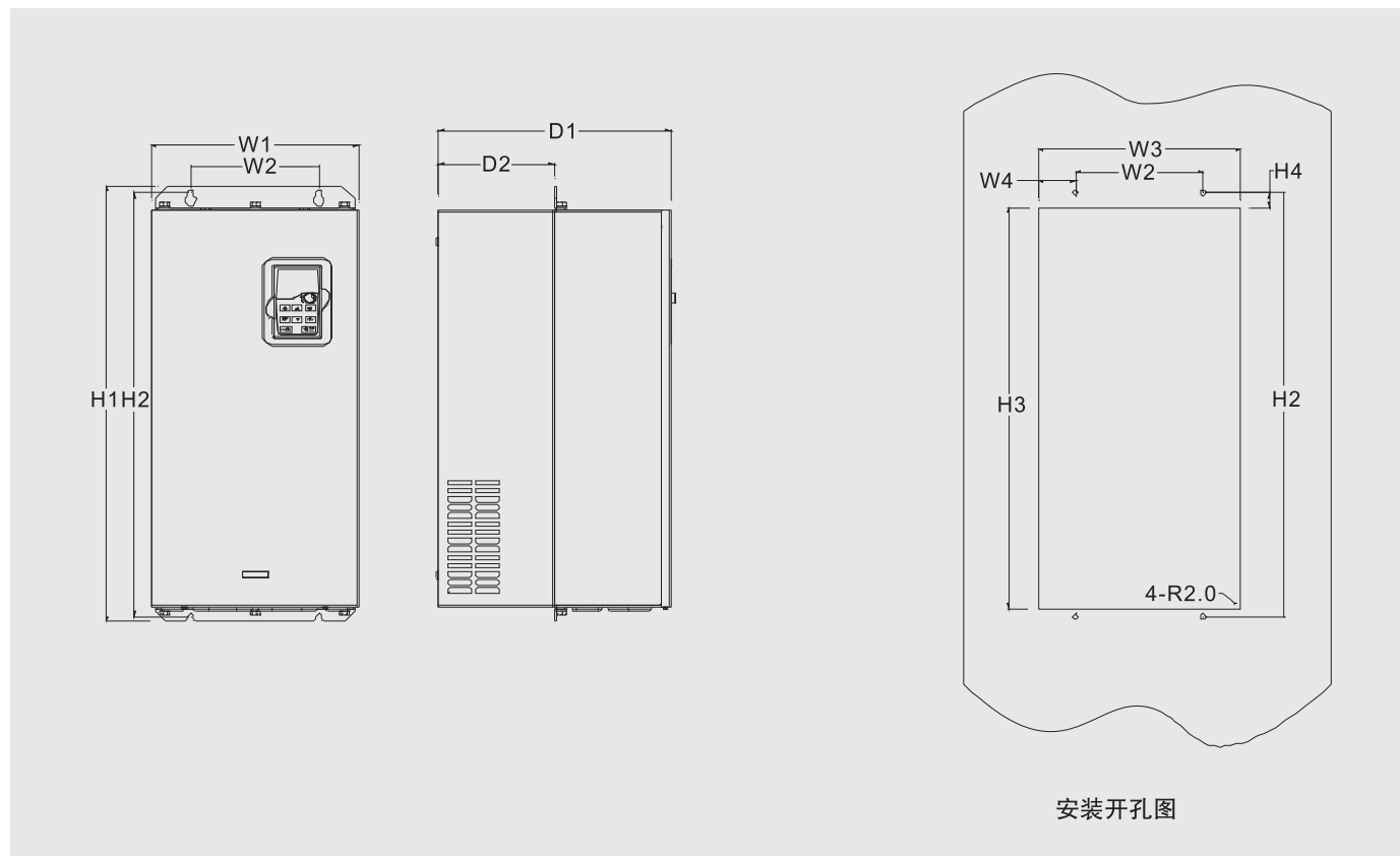
■ 380V 37~110kW ( 660V 22~132kW ) 法兰安装示意图
