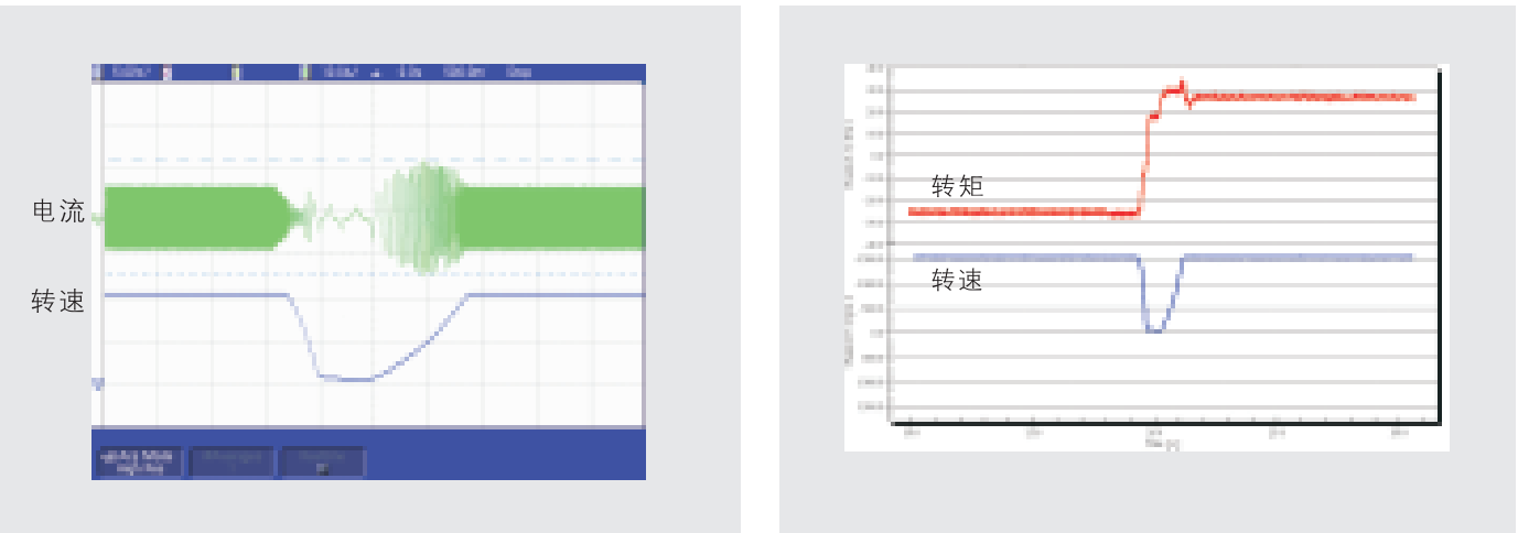
永磁同步电机转矩控制模式100Hz带100%额定负载正反转的电流、转矩与转速波形
