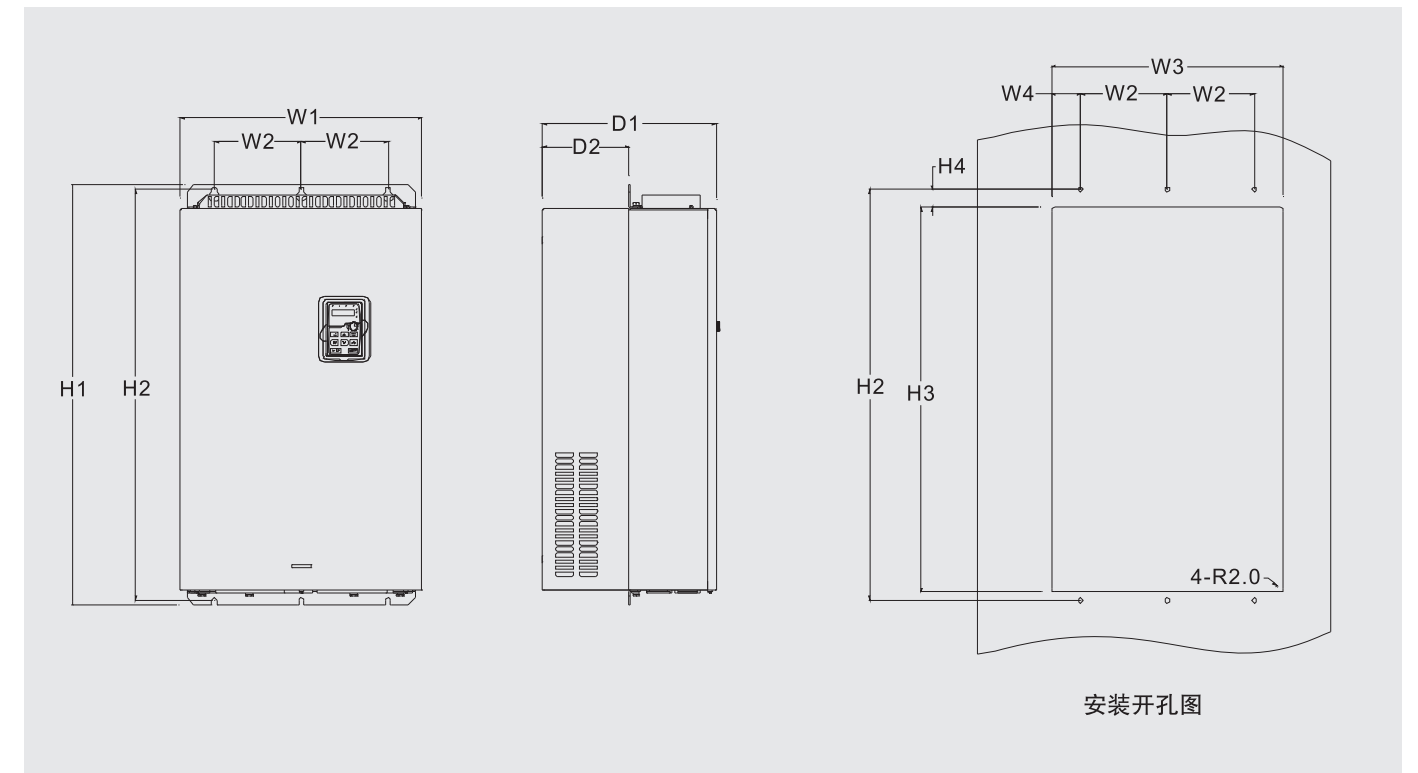
■ 380V 132~200kW ( 660V 160~220kW ) 法兰安装示意图
