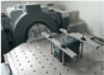
电动振动系统
