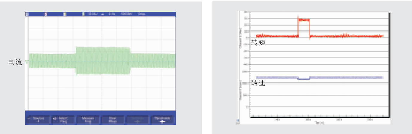
异步电机转矩控制模式带100%额定负载突然加载和卸载的电流、转矩与转速波形
